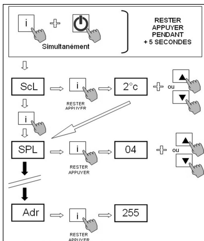
Fig. 5 Réglage des paramètres (Voir liste)
