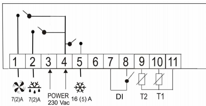
Fig. 7 Schéma de câblage
