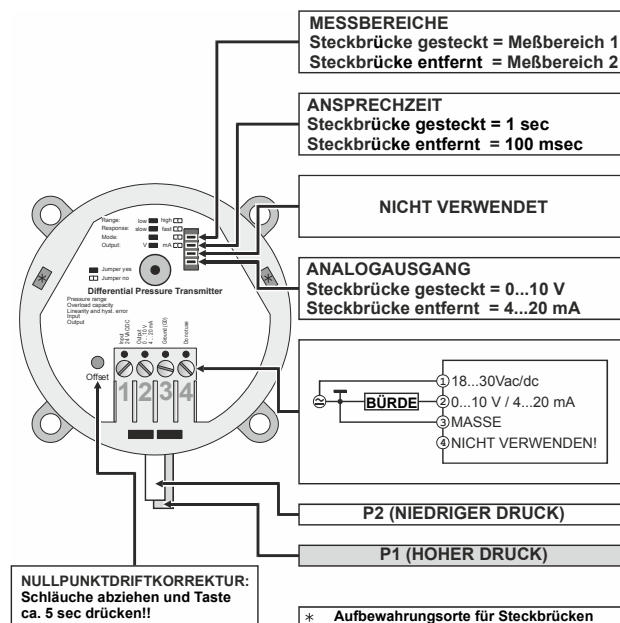
Abb. 3. Elektrischer Anschluß
