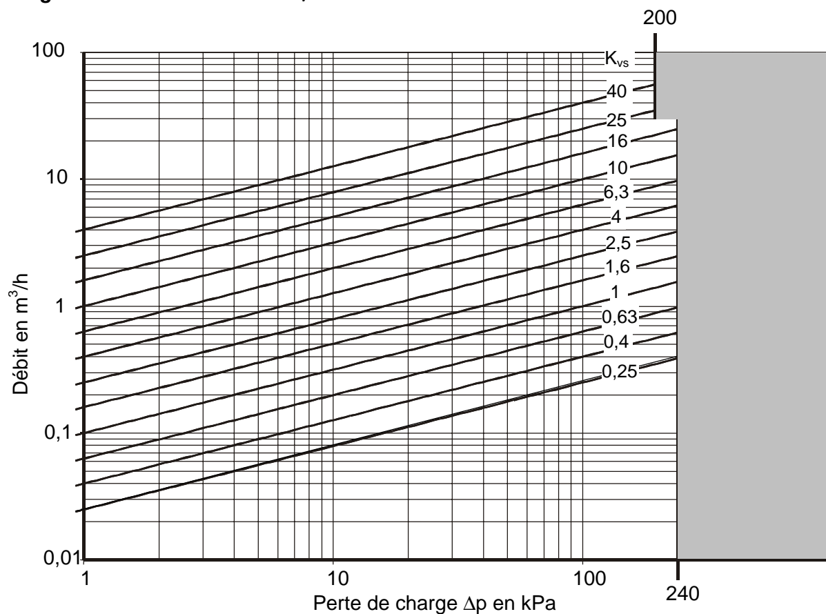
Diagramme de sélection des k_v
