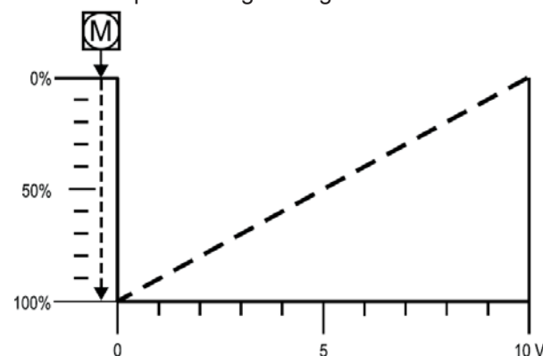
Figure 6 : Action inverse L'axe se rétracte quand le signal augmente.
