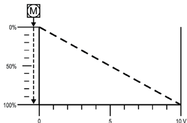
Figure 5 : Action directe L'axe s'étend quand le signal augmente.
