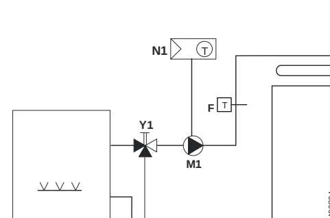
Thermostat d'ambiance avec régulation directe d'un système hydraulique de chauffage par le sol.
